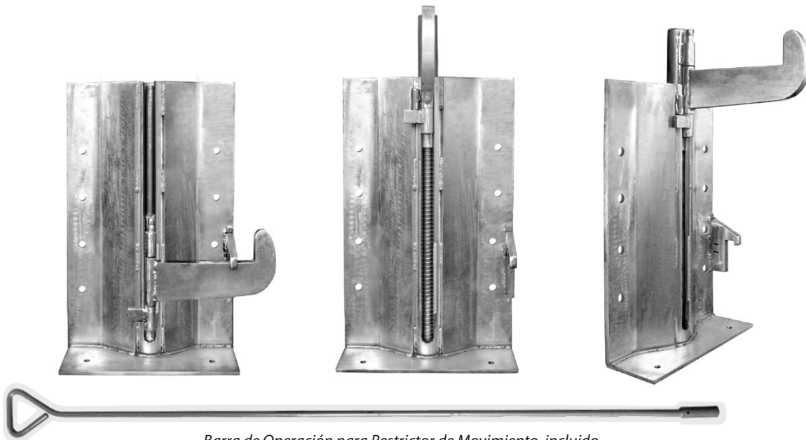
Barra de Operación para Restrictor de Movimiento, incluido.
